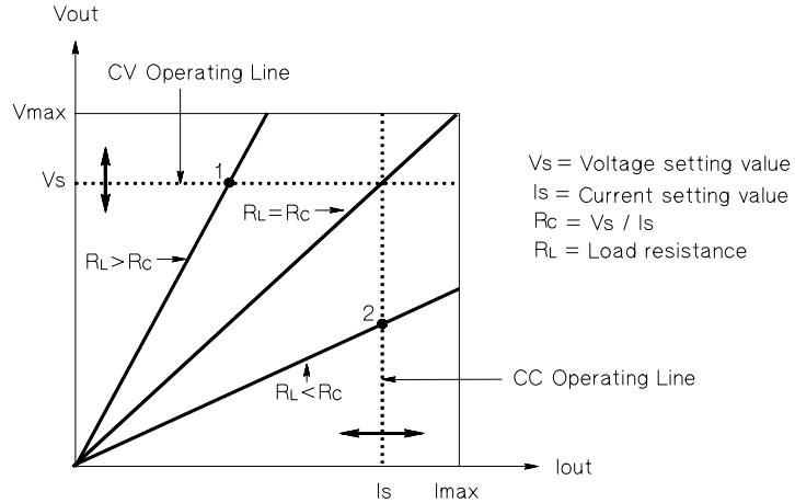
그림 7-5. 출력 특성
