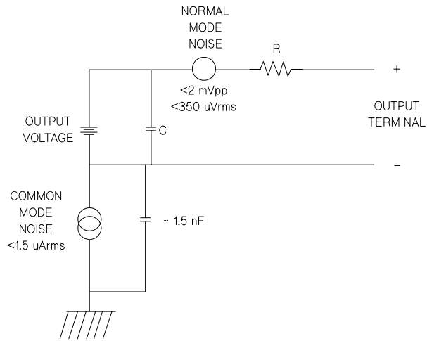
그림 7-6. 공통 모드 및 정상 모드 잡음원의 개략도
