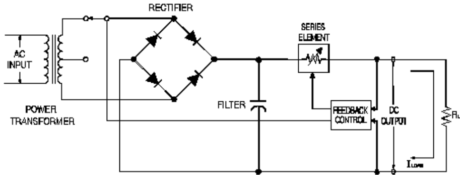
그림 7-5. 탭 선택 기능이 있는 간단한 직렬 레귤레이션 전원공급기의 다이어그램
