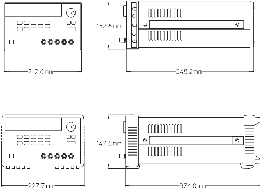
그림 8-1. Agilent E3632A 전원공급기의 치수
