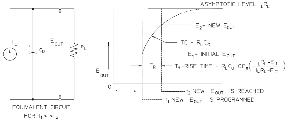
그림 7-8. 응답 속도 - 상향 프로그래밍 (최대 부하)
