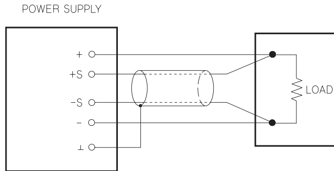
그림 3-2. 원격 전압 감지 연결
